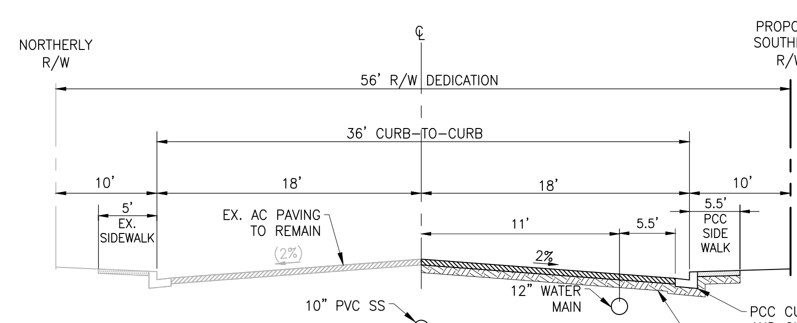
SECTION - S. OCEANSIDE BLVD. ADJACENT TO NCTD PROPERTY STA 11+24.66 - 17+41.17 SCALE: N.T.S.
