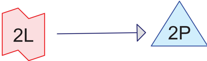
BMP-2 100-YR
