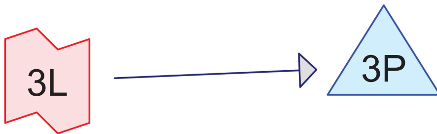
BMP-3 100-YR
